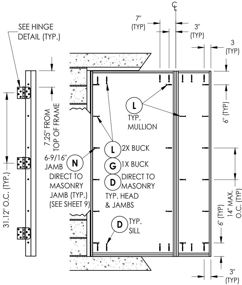
HINGE JAMB
